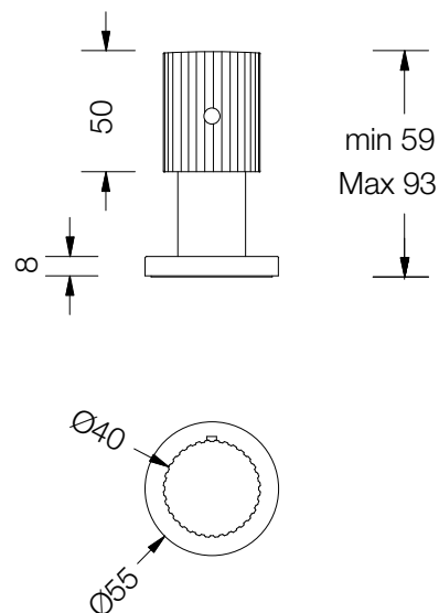
DISEGNO - DRAWING
