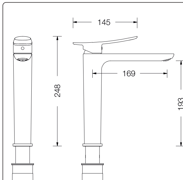
DISEGNO - DRAWING
