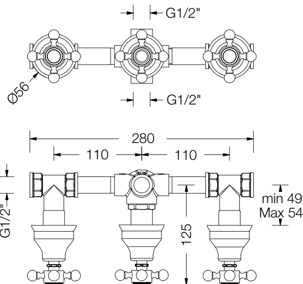
DISEGNO - DRAWING
