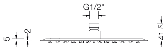
DISEGNO - DRAWING
