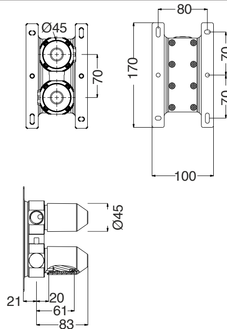
DISEGNO - DRAWING
