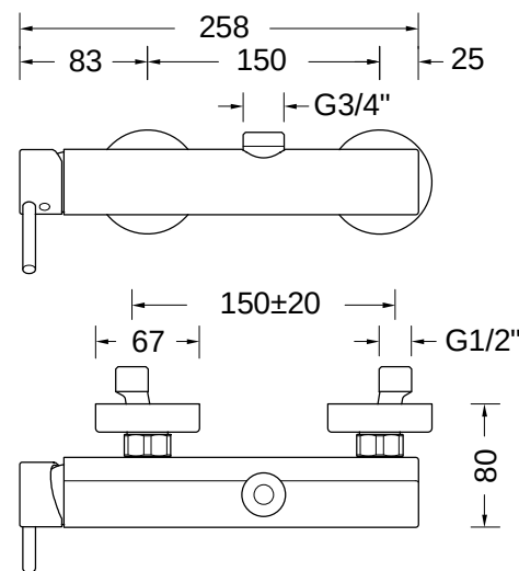
DISEGNO - DRAWING 711000
