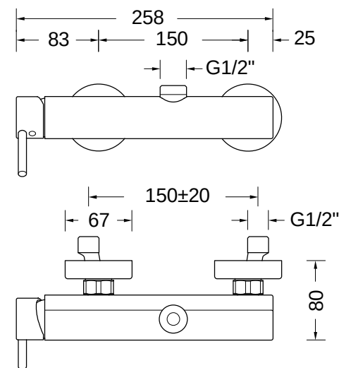
DISEGNO - DRAWING 711000B
