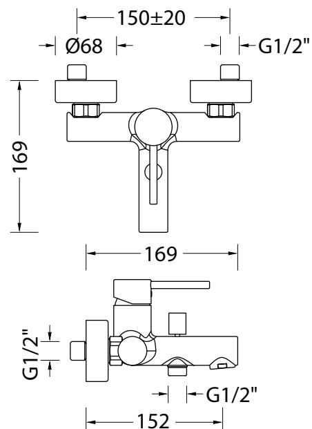
DISEGNO - DRAWING
