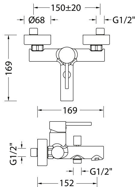
DISEGNO - DRAWING
