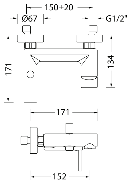
DISEGNO - DRAWING
