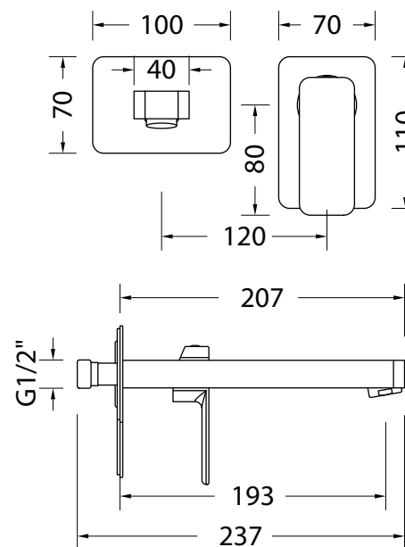
DISEGNO - DRAWING
