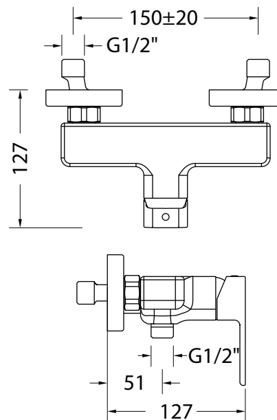
DISEGNO - DRAWING
