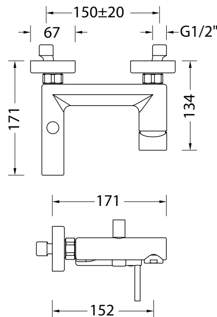
DISEGNO - DRAWING
