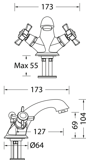
DISEGNO - DRAWING
