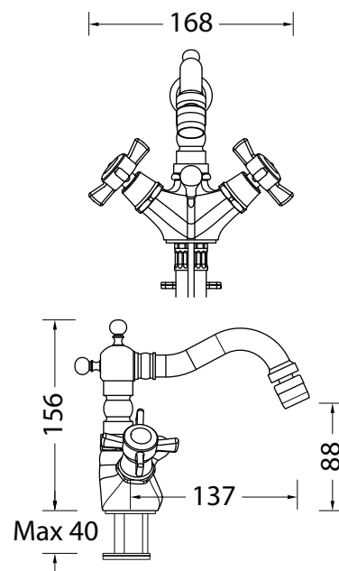
DISEGNO - DRAWING
