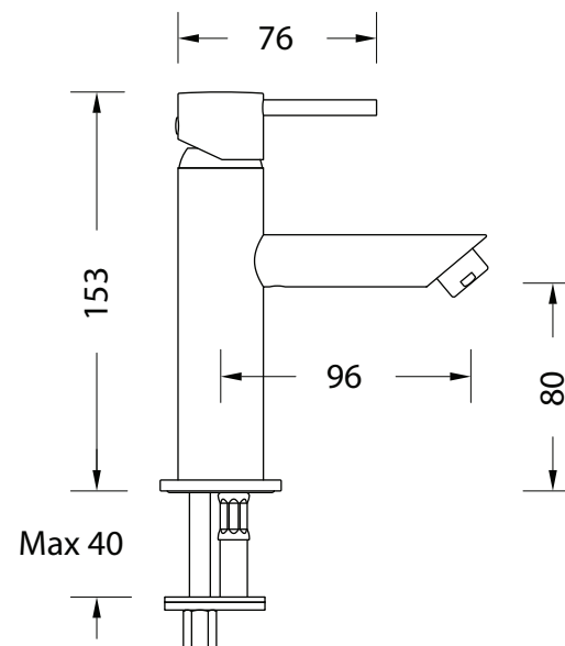
DISEGNO - DRAWING
