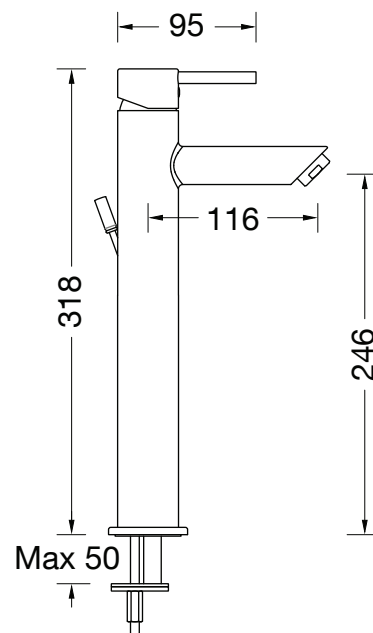
DISEGNO - DRAWING
