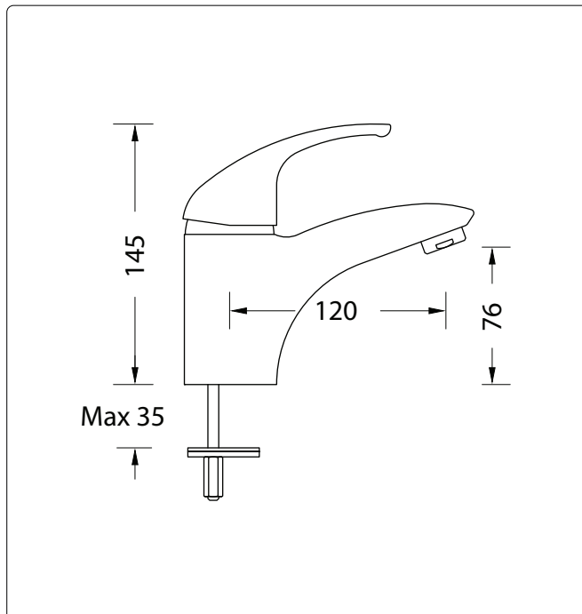
DISEGNO - DRAWING
