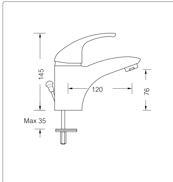
DISEGNO - DRAWING
