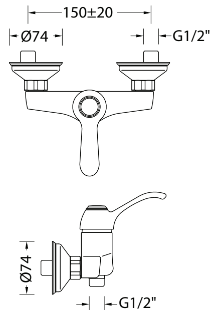
DISEGNO - DRAWING
