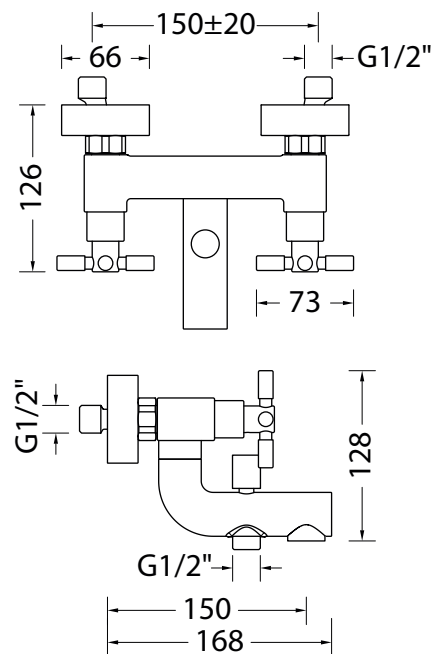
DISEGNO - DRAWING
