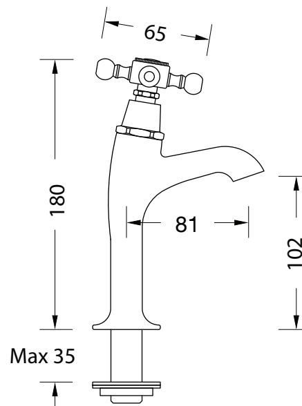
DISEGNO - DRAWING
