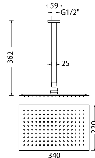
DISEGNO - DRAWING R51931
