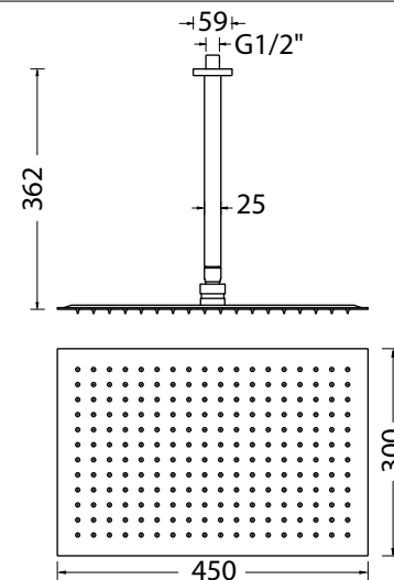
DISEGNO - DRAWING R51932
