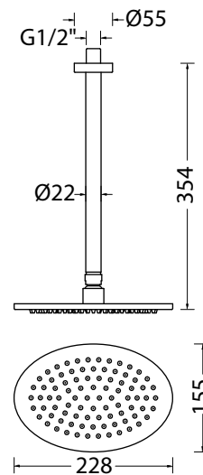
DISEGNO - DRAWING R51906
