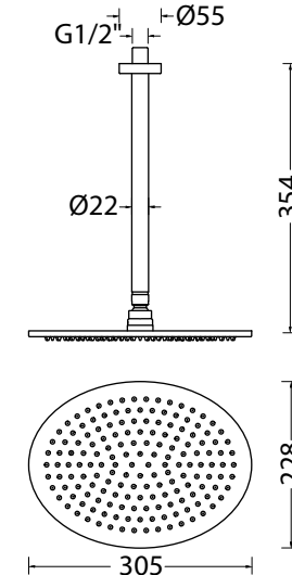
DISEGNO - DRAWING R51907
