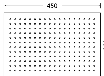
DISEGNO - DRAWING R50030
