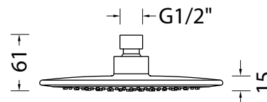
DISEGNO - DRAWING
