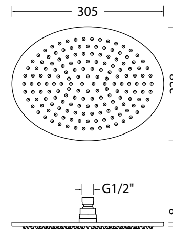
DISEGNO - DRAWING R50007
