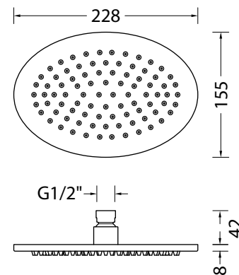
DISEGNO - DRAWING R50006
