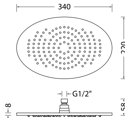
DISEGNO - DRAWING R50013
