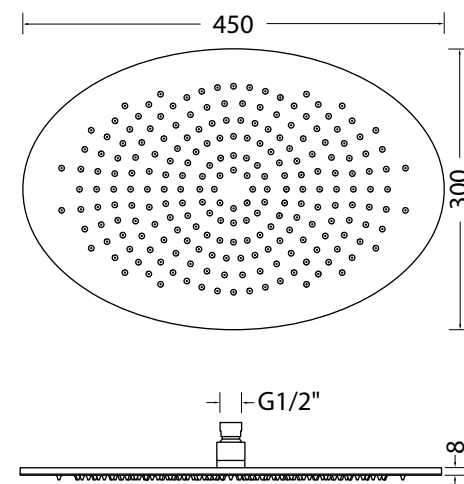
DISEGNO - DRAWING R50014
