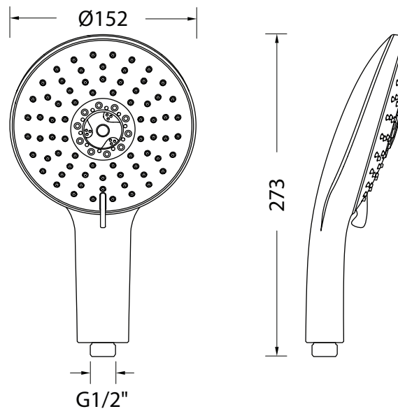
DISEGNO - DRAWING
