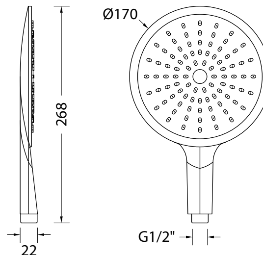
DISEGNO - DRAWING
