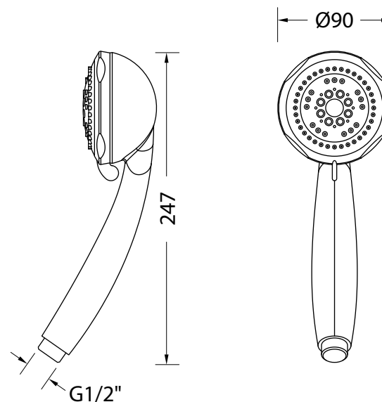
DISEGNO - DRAWING
