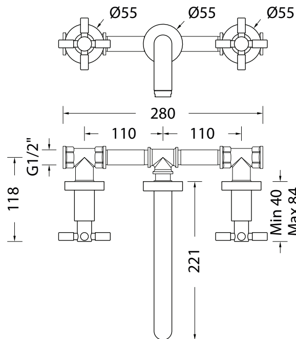
DISEGNO - DRAWING
