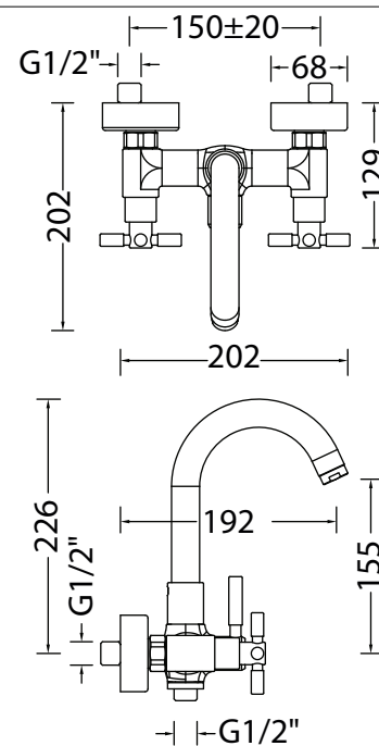
DISEGNO - DRAWING
