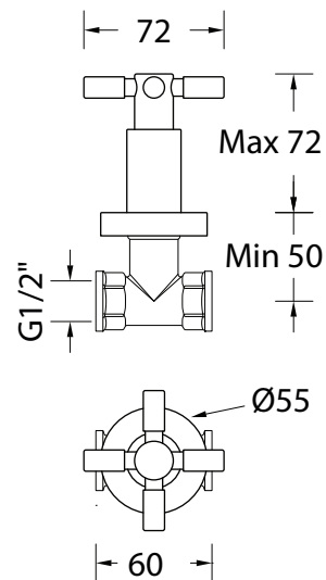
DISEGNO - DRAWING
