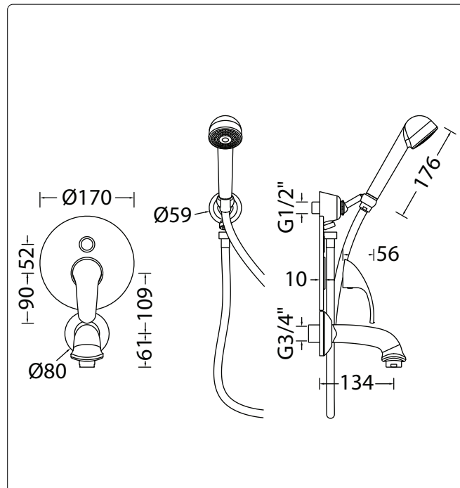
DISEGNO - DRAWING
