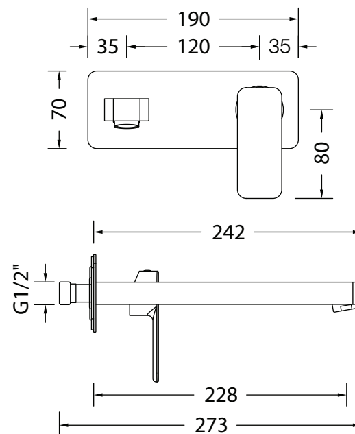
DISEGNO - DRAWING
