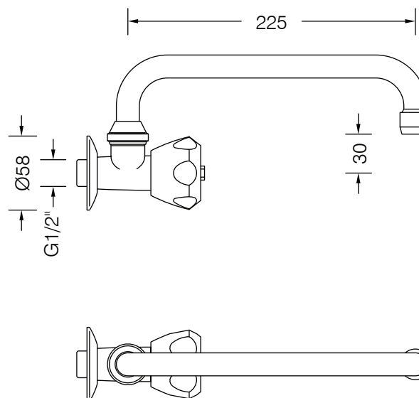
DISEGNO - DRAWING
