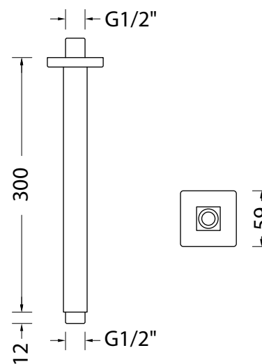
DISEGNO - DRAWING R50807
