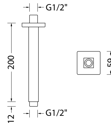
DISEGNO - DRAWING R50806
