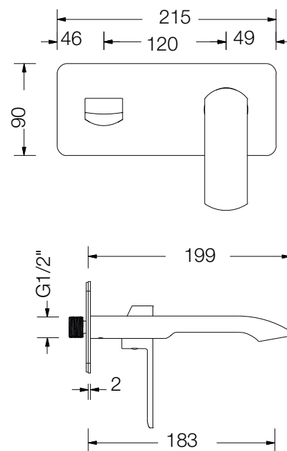
DISEGNO - DRAWING
