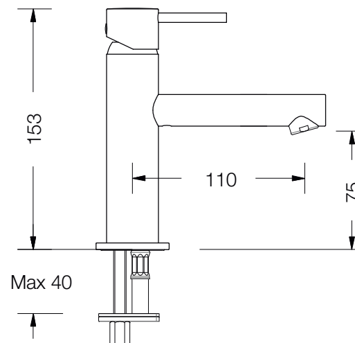
DISEGNO - DRAWING
