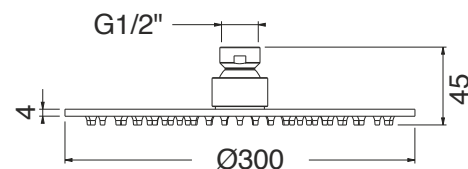
DISEGNO - DRAWING
