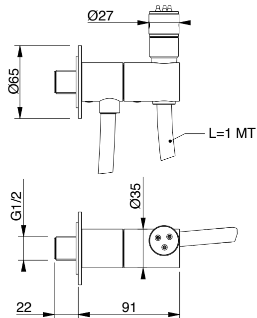
DISEGNO - DRAWING
