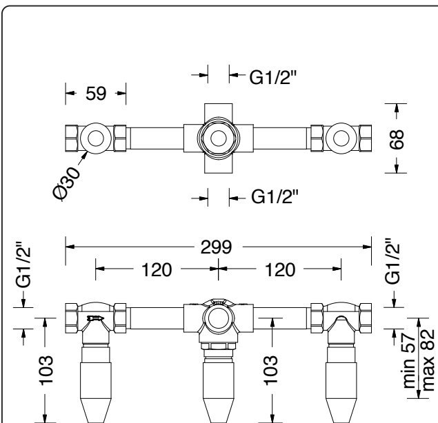
DISEGNO - DRAWING
