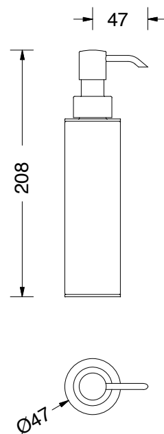
DISEGNO - DRAWING
