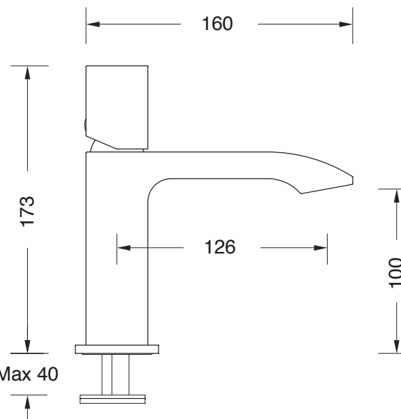
DISEGNO - DRAWING
