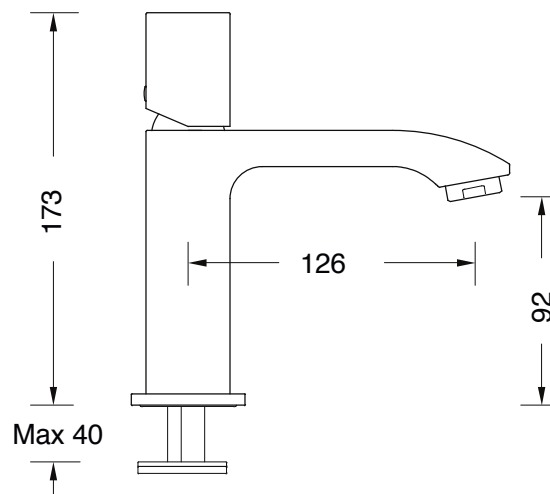
DISEGNO - DRAWING
