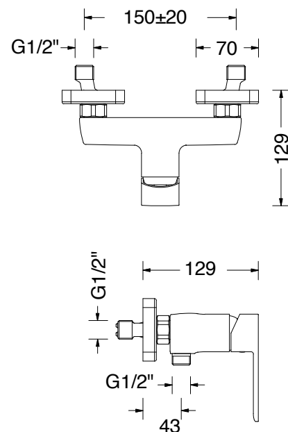
DISEGNO - DRAWING
