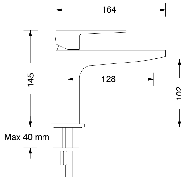
DISEGNO - DRAWING
