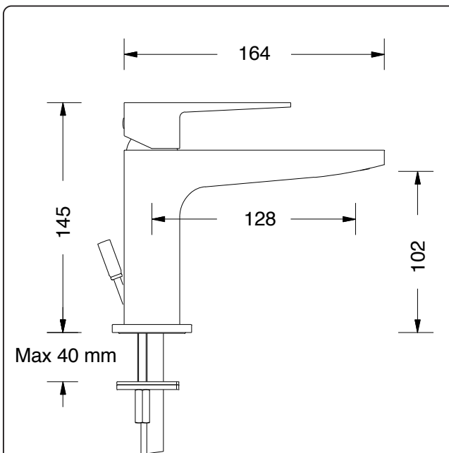
DISEGNO - DRAWING
