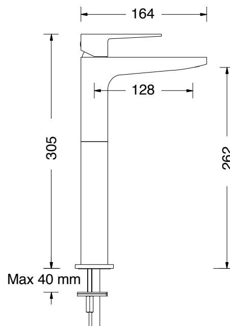
DISEGNO - DRAWING
