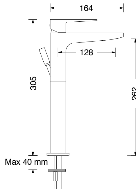
DISEGNO - DRAWING
