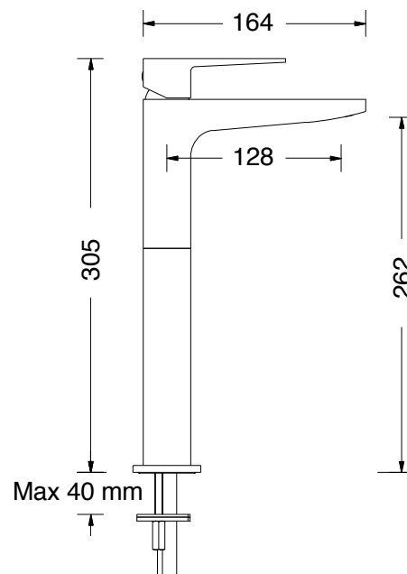
DISEGNO - DRAWING
